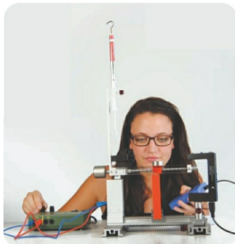
A centrifugális erő függése a szögsebességtől
