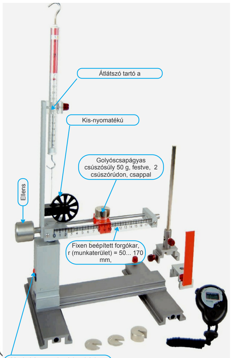
A centrifugális erő függése a tömegtől
