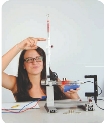
A centrifugális erő függése a forgási sugártól
