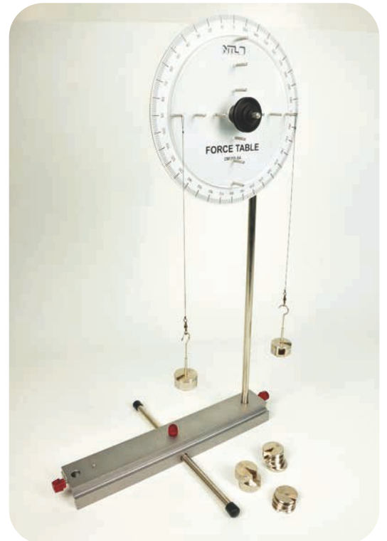
Forgató nyomatékok egyensúlya
