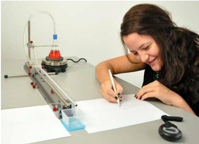
TDS 1.4. Szilárd anyagok lineáris hőtágulása
